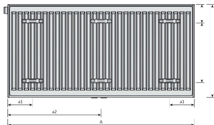
Baksida (modell Flex 21S, 22 och 33)
